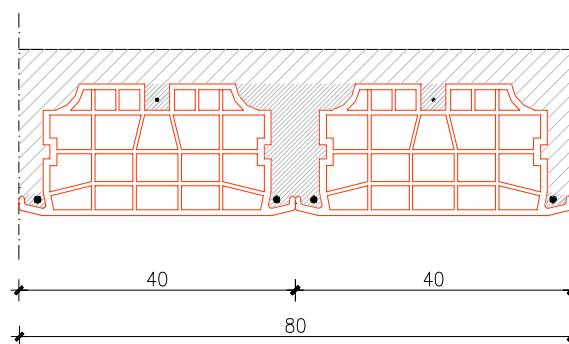
Interasse ridotto
